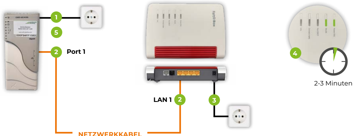
Netzabschlussgerät (ONT, z. B. GENEXIS-Box)
